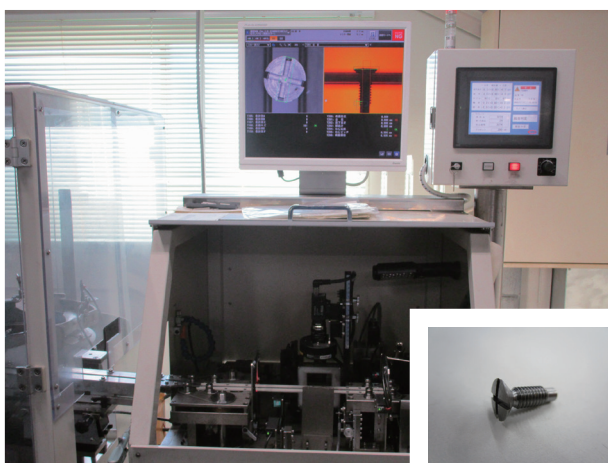
加工された精密ネジ・特殊ネジの画像処理による寸法検査。
